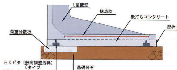
参考施工断面図
