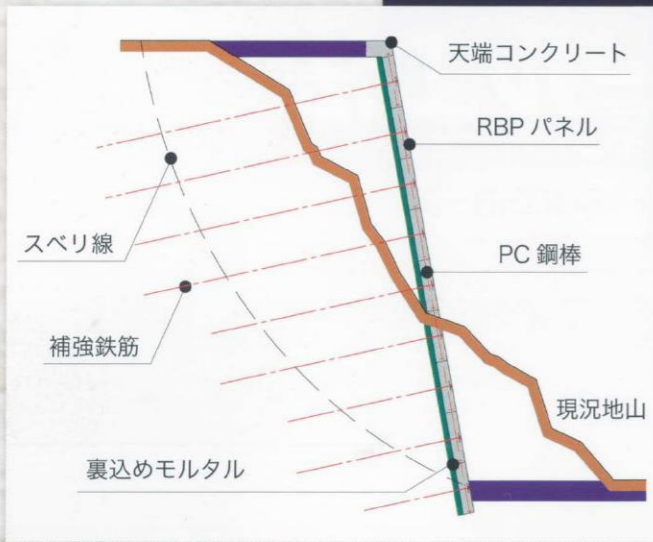
■参考断面図
