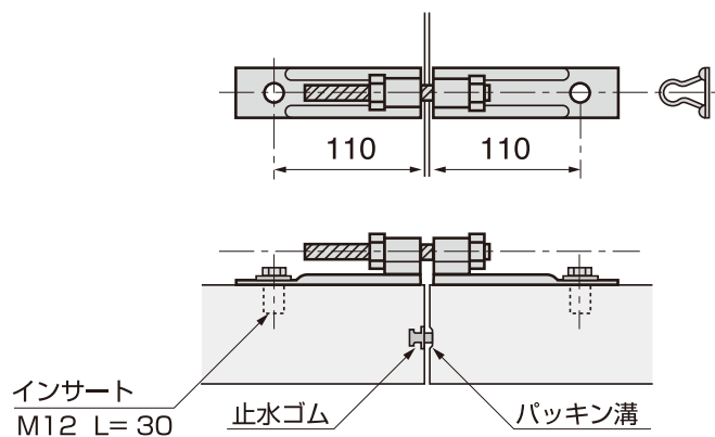
連結詳細図
