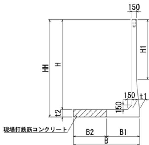
標準断面図
