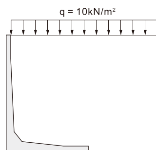
ケース B：載荷重を底版上に載荷する場合
