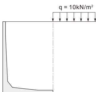
ケース A：載荷重を底版上に載荷しない場合
