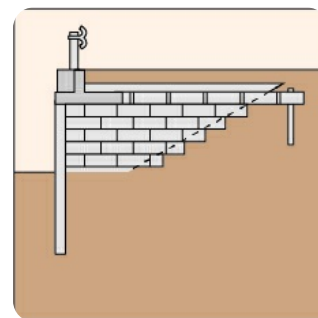
軽量盛土
